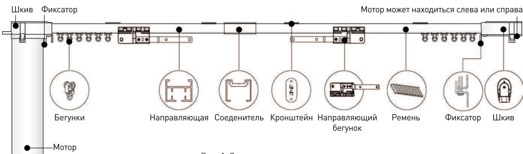
Рис. 1. Состав комплекта
